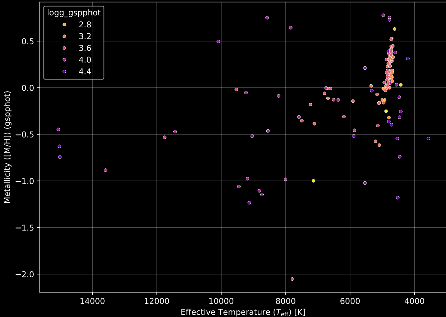
APOGEE DR17 Field: [060+00_btx] Stellar Population Parameters (n= 136)
